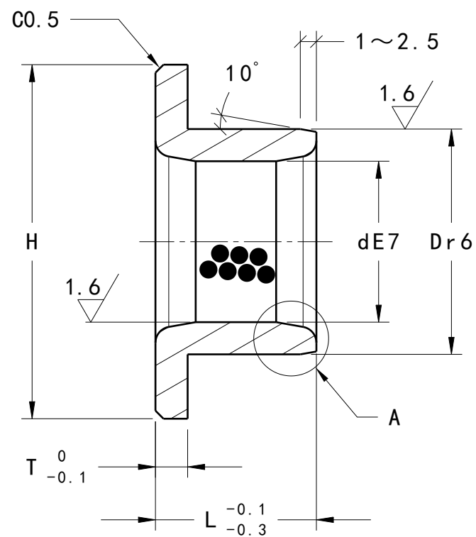
Section view A-A Scale: 3:1
