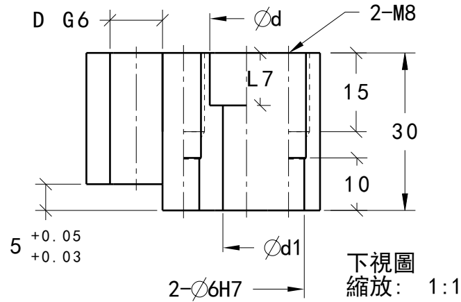
前視圖 縮放: 1:1
