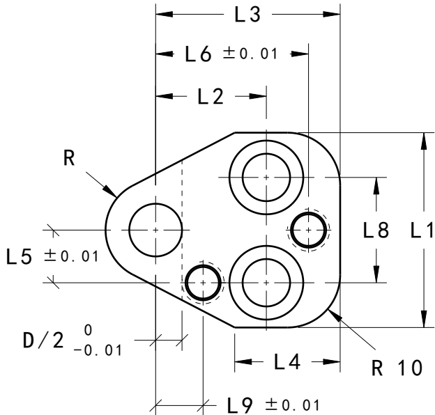
前視圖 縮放: 1:1
